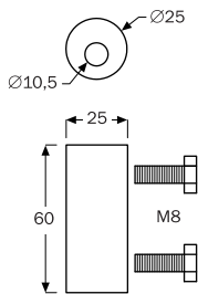
Modelo Unión lineal 50 x 50 mm 2
