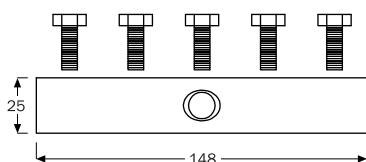
Modelo Unión en Cruz
