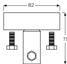
Modelo Unión en 'T' (2 piezas)
