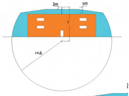
Fig. 3 – Volume protégé par un paratonnerre PDA
